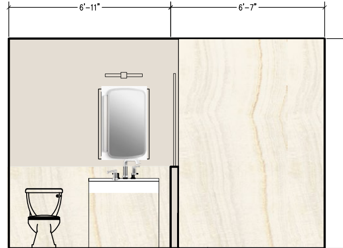
ELEVATION B
