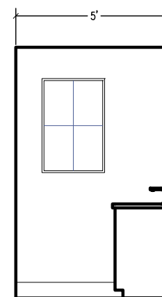
ELEVATION B
