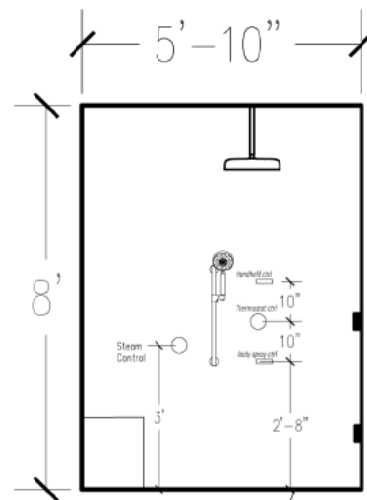
ELEVATION A
