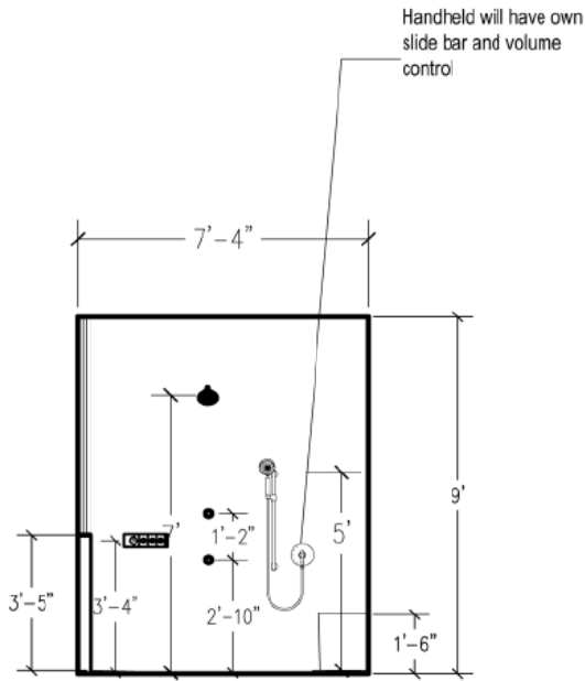
ELEVATION A
