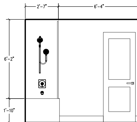
ELEVATION A
