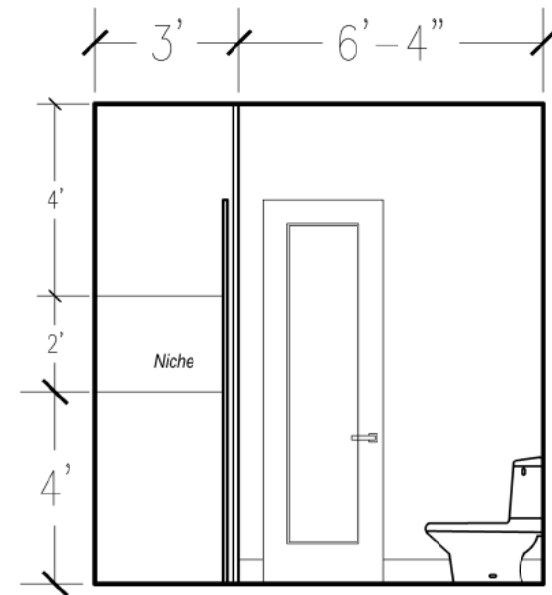
ELEVATION B
