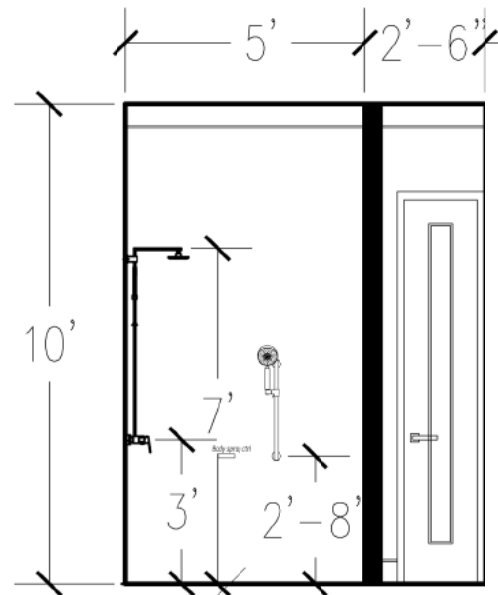
ELEVATION A
