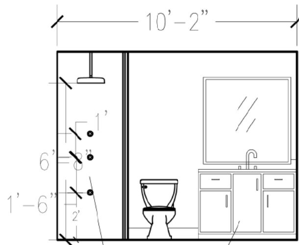
ELEVATION B
