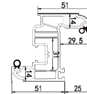
65 inward sash
