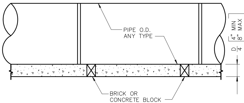
LONGITUDINAL SECTION
