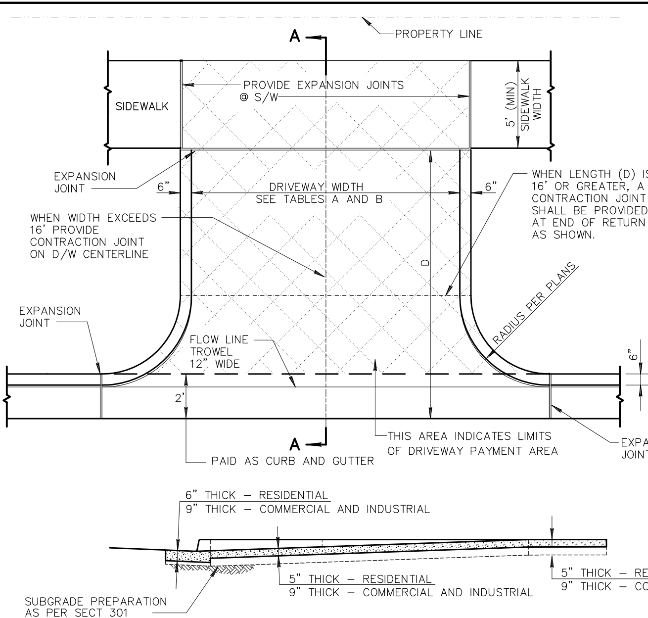
SECTION A-A
