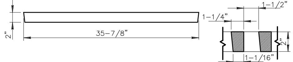
SECTION A-A
