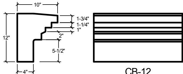
CB-12 L&R Returns 42" length
