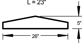
WC - 24 TE = 36" L = 23"
