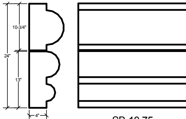
SB-10.75 L&R Returns 24" length
