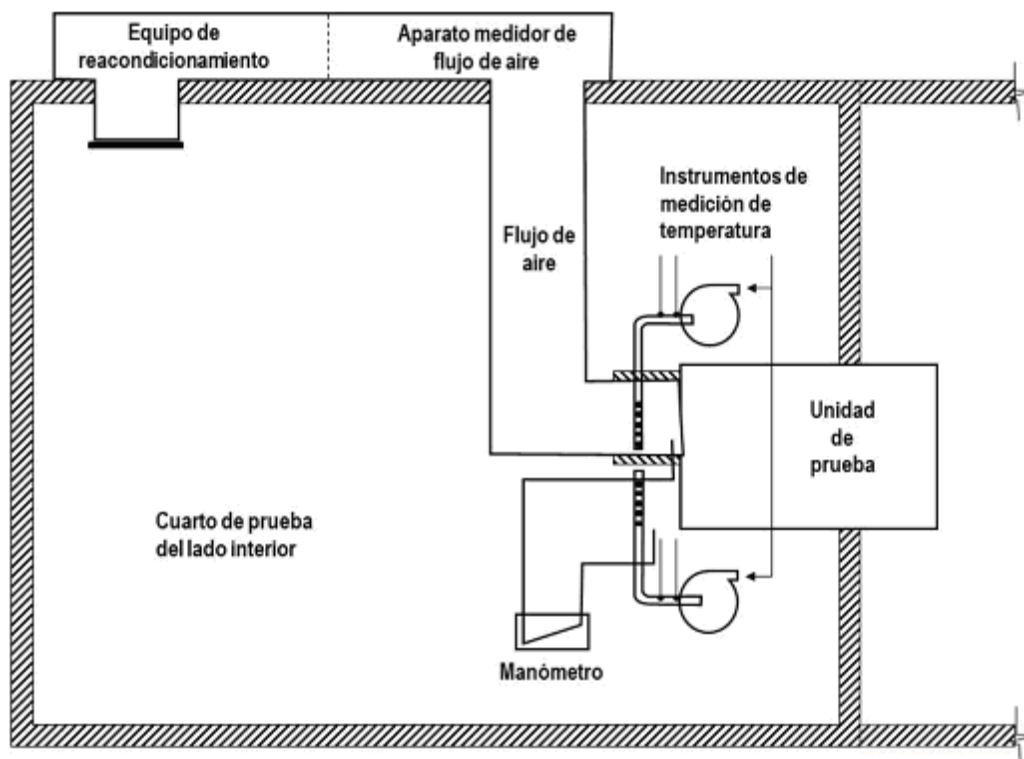
Figura A.4-Cuarto de aire-entalpía
