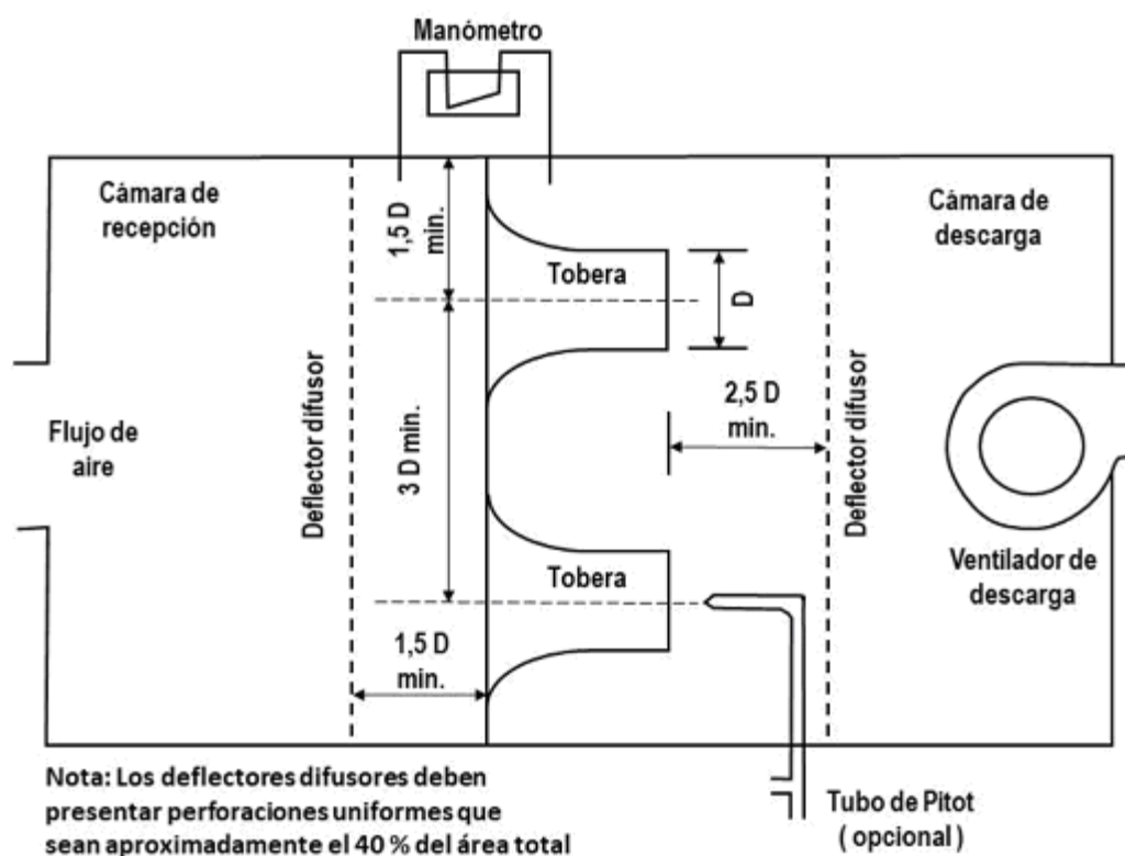
Figura A.5-Aparato de medición de flujo de aire
