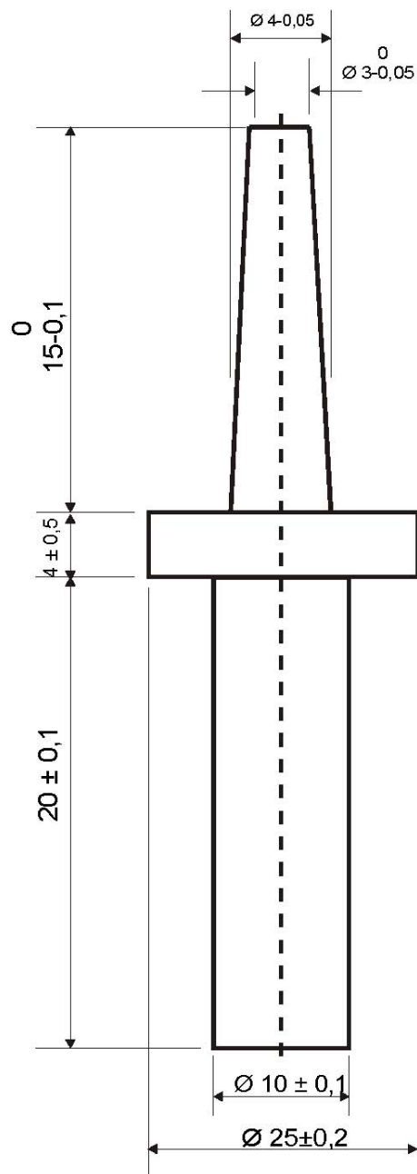
Figura 2. Aguja de prueba
