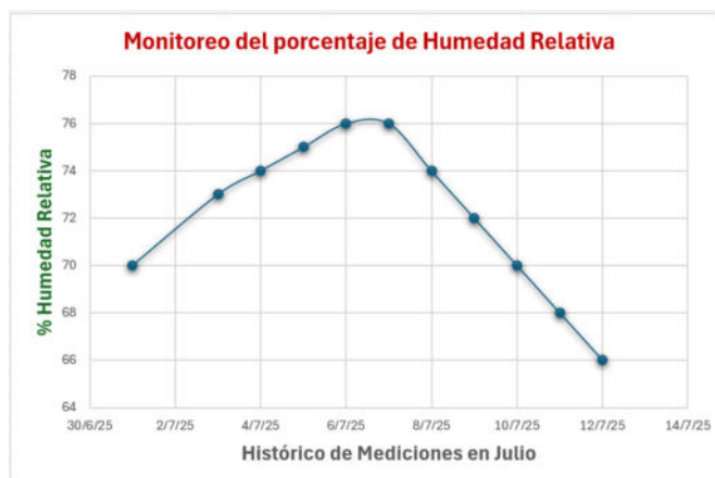
Figura 3. Historial de datos capturados del monitoreo del porcentaje de Humedad relativa.
