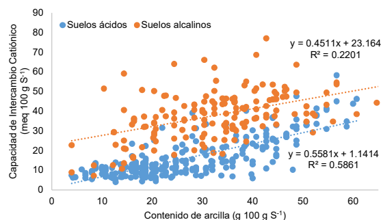
Figura 1a. Relación entre el contenido de arcilla y la CIC.
