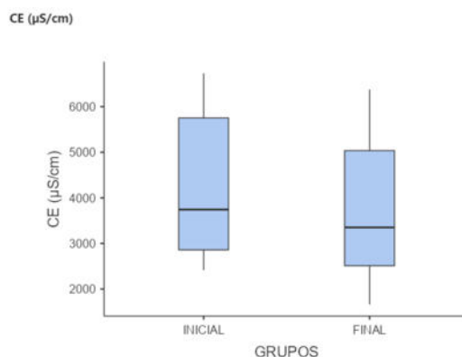
Figura 1. Gráfica de caja de la conductividad eléctrica ( \mu\text{S/cm} ) antes y después del tratamiento.
