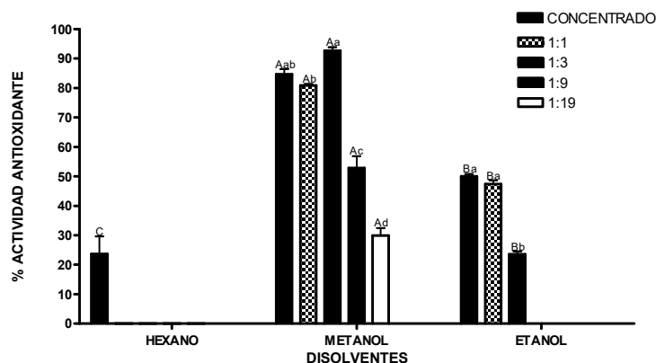
Figura 1. Resultados de la evaluación del potencial antioxidante con el radical libre DPPH en Chenopodium berlandieri .
