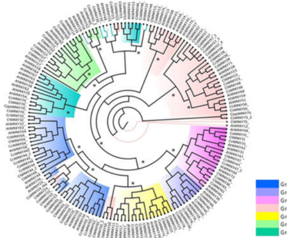
Figura 1. Consenso estricto de la filogenia de máxima parsimonia de los genes WRKY de Citrus latifolia (CIWRKY), C. sinensis (CsWRKY), C. clementina (CcWRKY) y Arabidopsis thaliana (AtWRKY). Los asteriscos indican un porcentaje de bootstrap/jackknife de 100/100.
