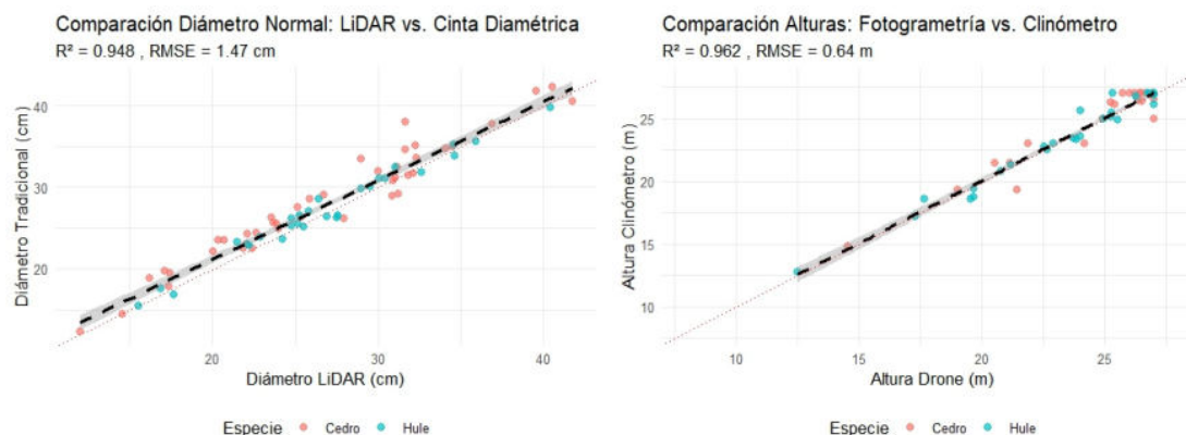
Figura 2. Comparación entre mediciones de DN y altura total mediante sensores remotos (LiDAR y dron) y métodos tradicionales (cinta métrica y clinómetro).
