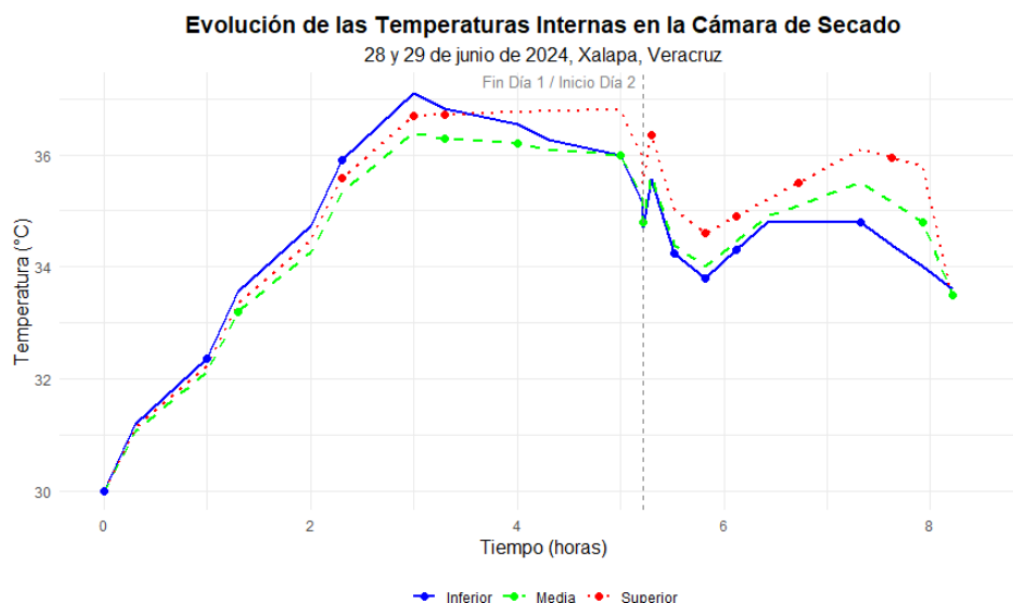
Figura 2. Temperaturas internas en la cámara de secado (28–29 de junio de 2024). La línea vertical en 5.22 h marca la transición entre días.
