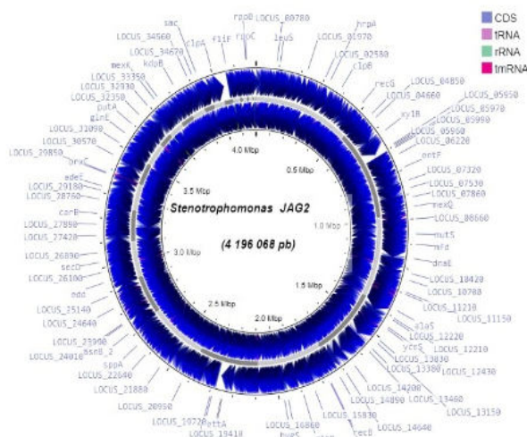
Figura 1. Mapa circular del genoma de Stenotrophomonas cepa JAG2. Se muestra la densidad de las regiones codificantes y la presencia de tRNA, rRNA y tmRNA.
