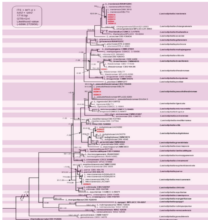
Figura 1. Árbol filogenético de Lasiodiplodia generado a partir del análisis de Máxima Verosimilitud del conjunto de datos concatenado de las regiones ITS, tef1-α , tub2 y rpb2 .
