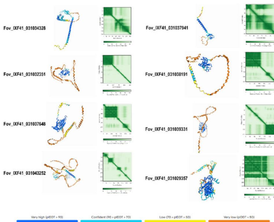
Figura 2. Estructura 3D predicha de las ocho proteínas efectoras asociadas a la patogenicidad, exclusivas de la cepa altamente virulenta Fov IXF41. El nivel de confianza en la predicción estructural se representa mediante una escala codificada por colores.
