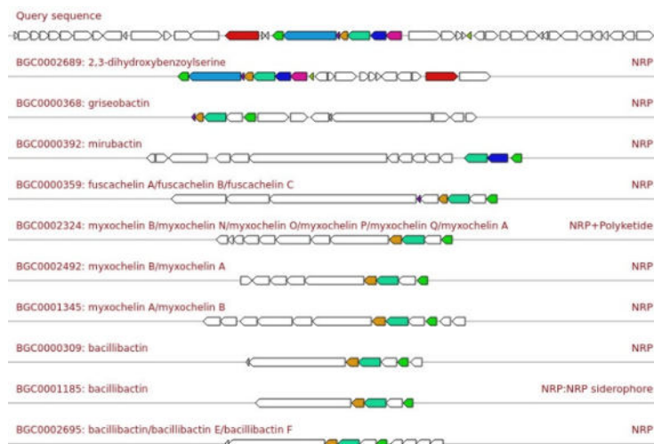
Figura 2. Comparación del BGC de biosíntesis de 2,3-dihidroxibenzoilserina en el genoma de Stenotrophomonas JAG2 con otros BGC conocidos.
