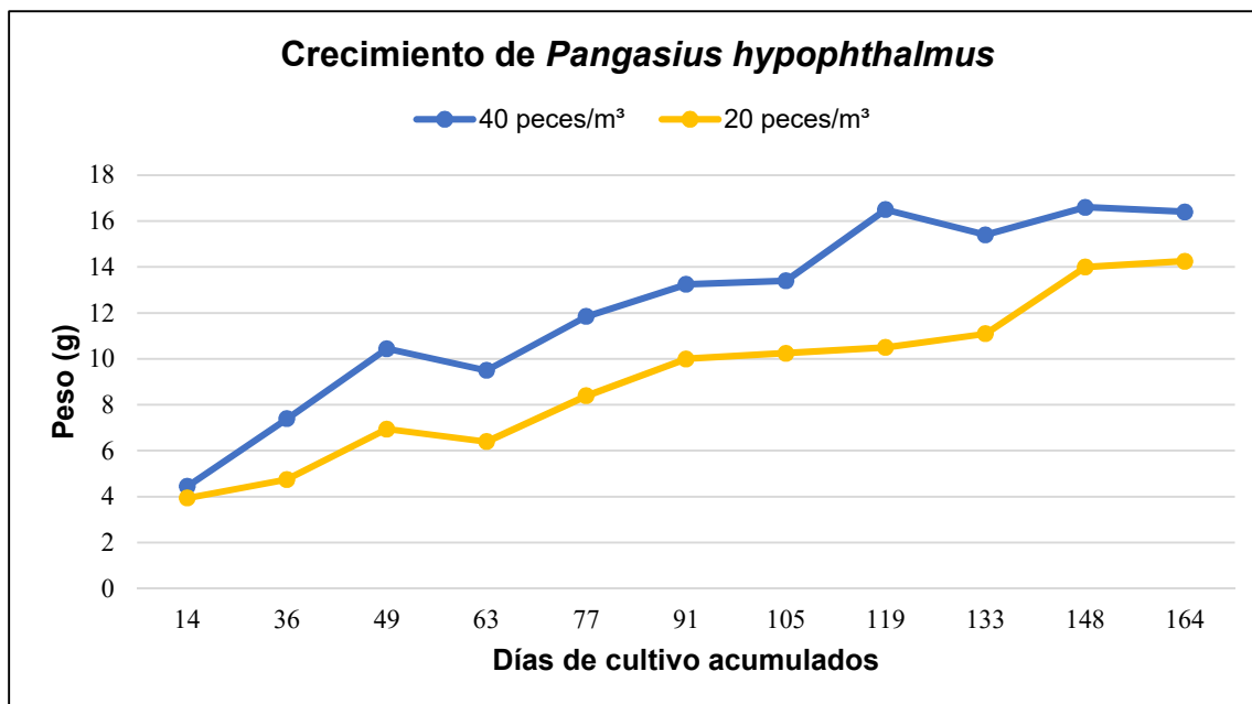
Figura 1. Evolución del peso promedio (g) de P. hypophthalmus bajo dos densidades de cultivo durante 164 días.
