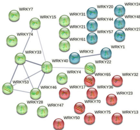
Figura 3. Red de co-expresión para 31 de las 32 proteínas CIWRKY en Citrus x latifolia en función de sus homólogos en Arabidopsis thaliana . El grosor y la intensidad de las líneas son proporcionales a la evidencia experimental de co-expresión entre proteínas en A. thaliana .
