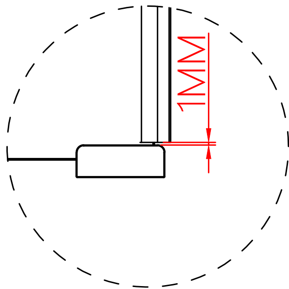
磁条安装位 与下滑块有1MM间隙
