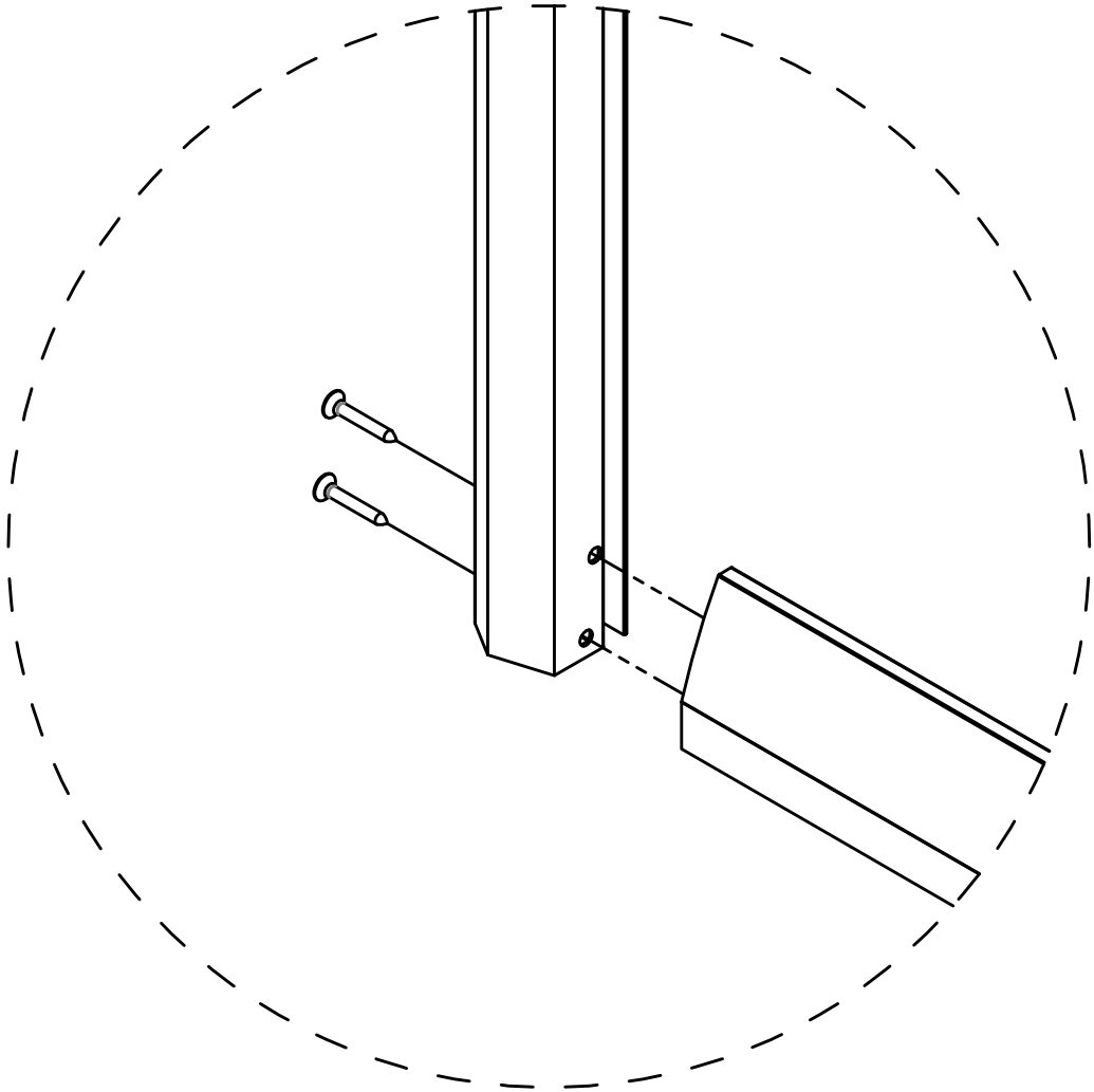
A处放大
