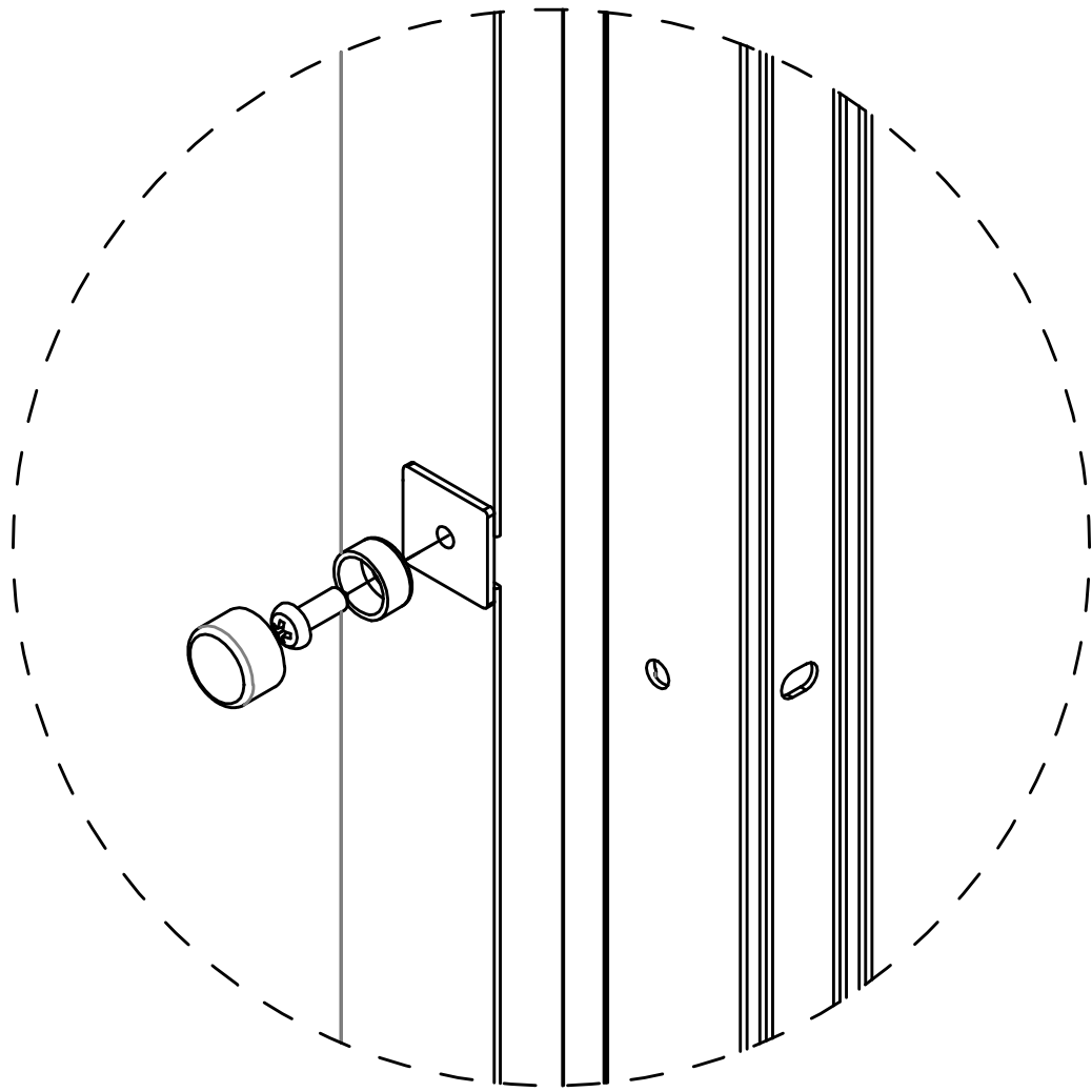
A处放大
