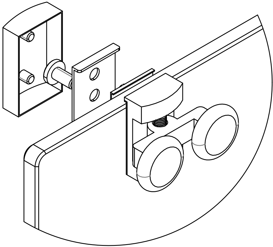
上轮
