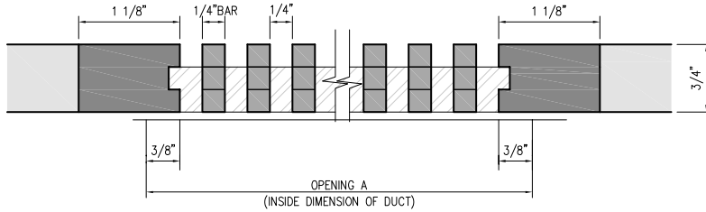
(M) SECTION DETAIL SCALE: 1'-0"=1'-0"
