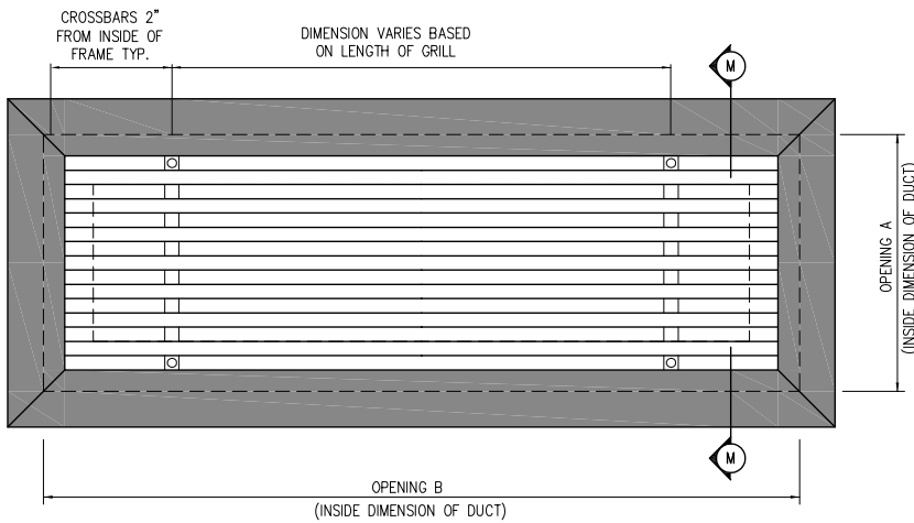
PLAN VIEW SCALE: 6"=1'-0"
