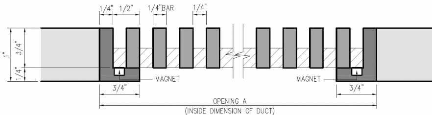
SECTION DETAIL SCALE: 1'-0"=1'-0"
