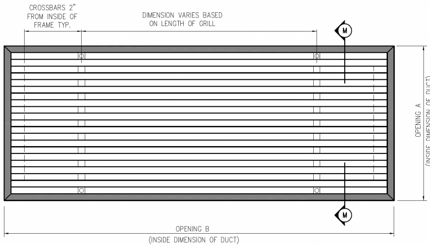
PLAN VIEW SCALE: 6"-0"=1'-0"
