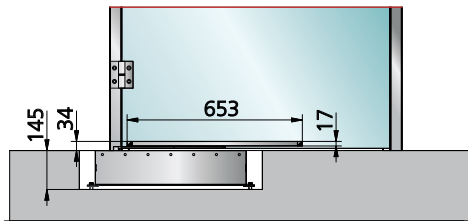
DIN left pulling function
