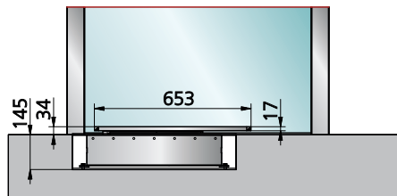
DIN right pushing function
