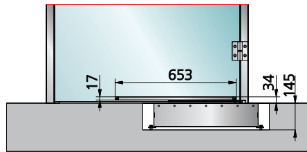
DIN right pulling function
