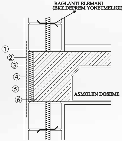
Şekil 4-Sandviç duvarlar
