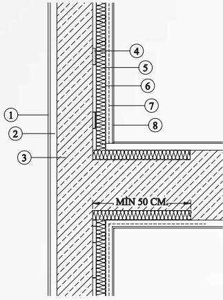
Şekil 3-Dış duvarların içten ısı yalıtımı
