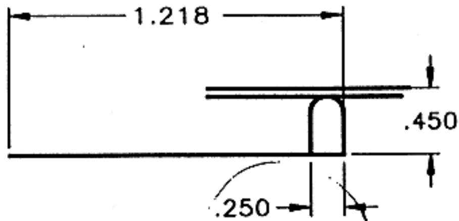
SLIDE STOP SLOT DTEAIL
