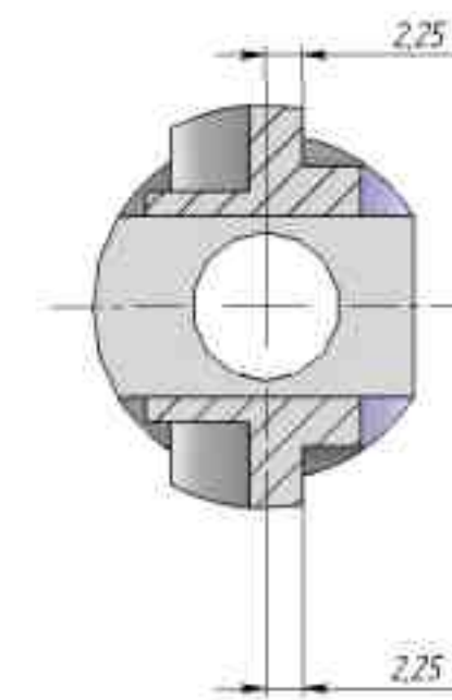
B-B (2 : 1)
