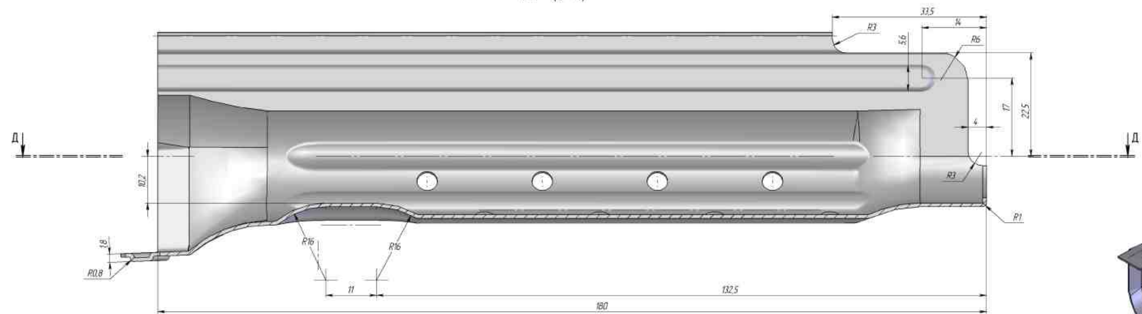
Г-Г (2 : 1)
