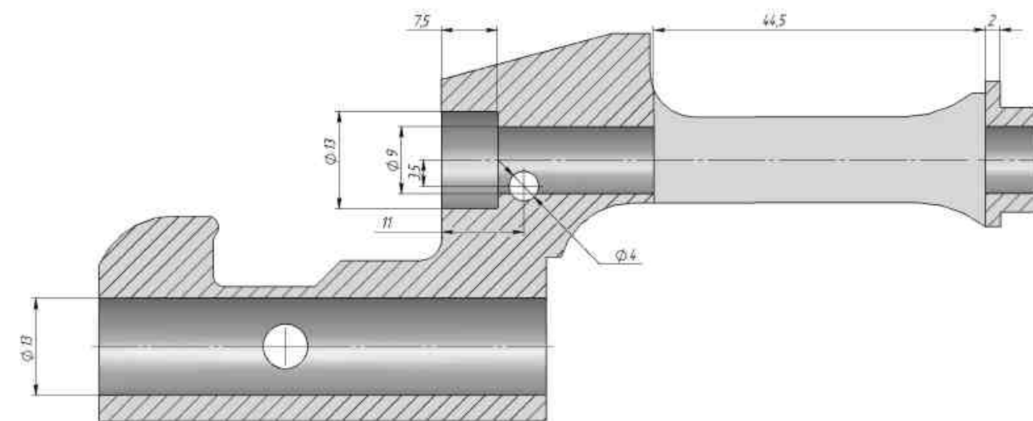
A-A (2 : 1)
