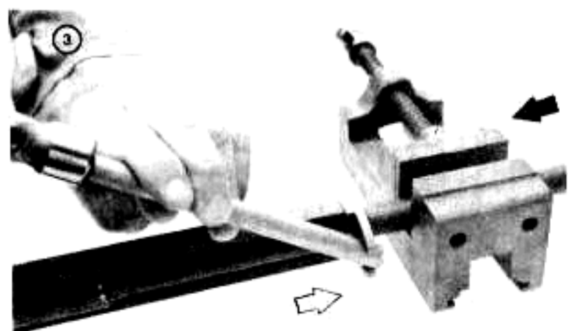
LOOSEN/TIGHTEN BAND
