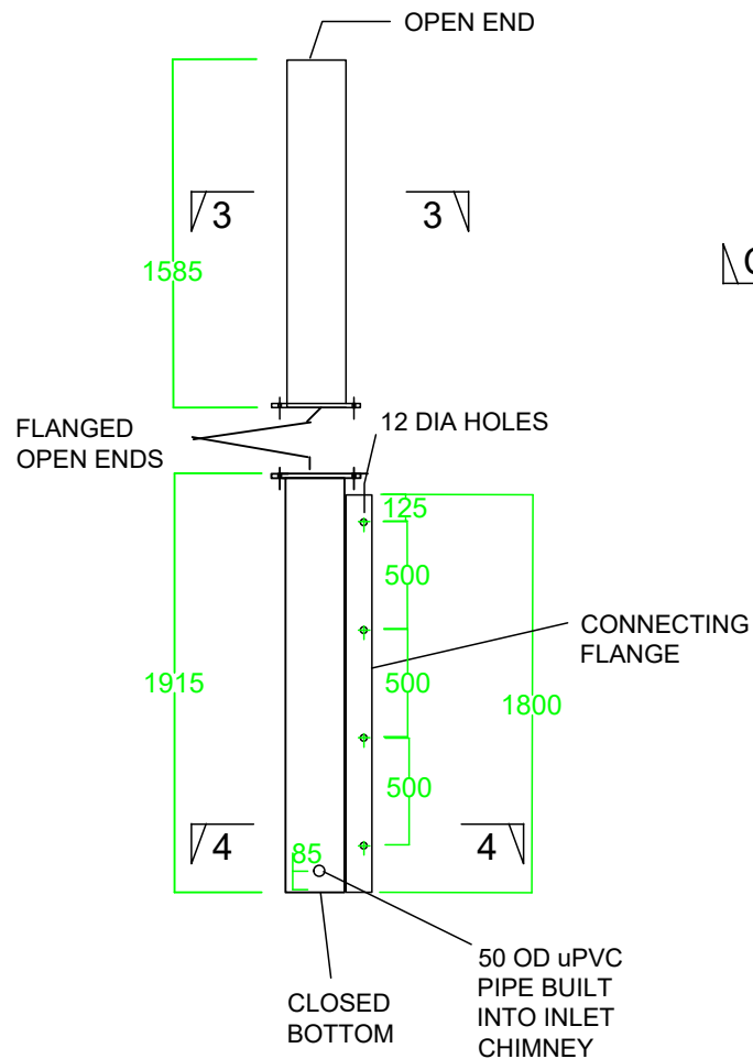
ELEVATION C-C
