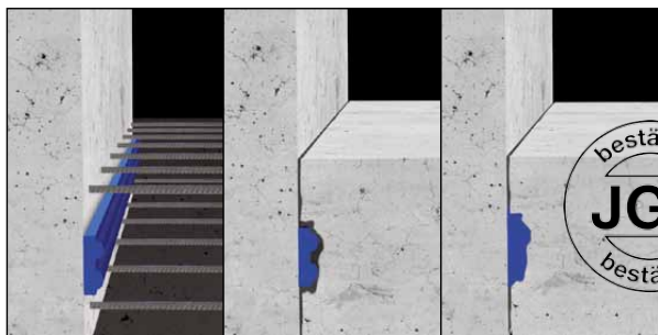
Medienbeständiges quellfähiges Dichtungs-System für Arbeitsfugen
