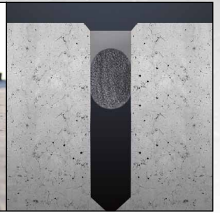
Fugenprofile und dauerelastische Dichtmasse zur Abdichtung von Dehnfugen, JGS-beständig
