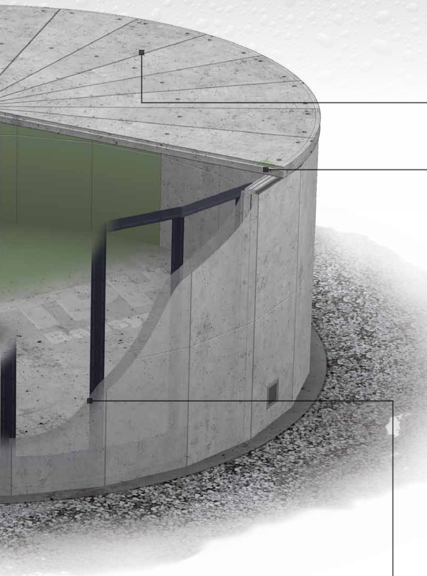
Fugenprofile und dauerelastische Dichtmasse zur Abdichtung von Dehnfugen, JGS-beständig
