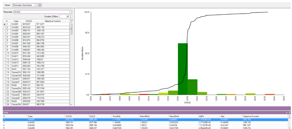
Parameter distribution
