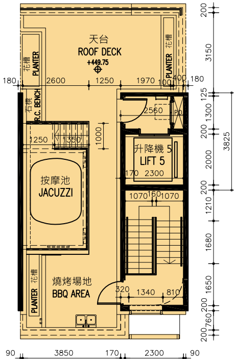
上層天台 UPPER ROOF AT LEVEL + 449.75
