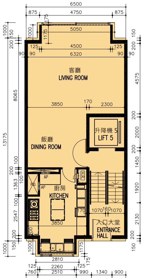
地下 GROUND FLOOR
