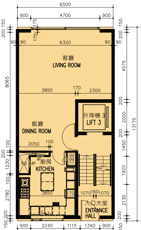
地下 GROUND FLOOR
