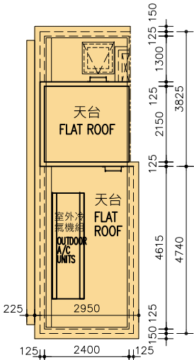
頂層天台 TOP ROOF
