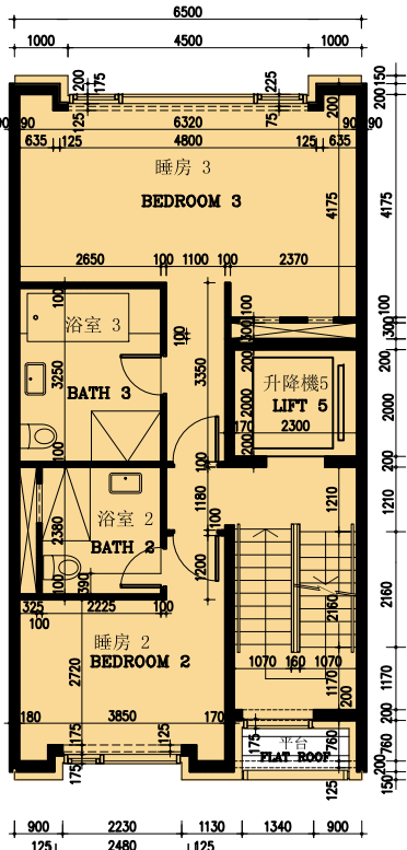
二樓 2ND FLOOR
