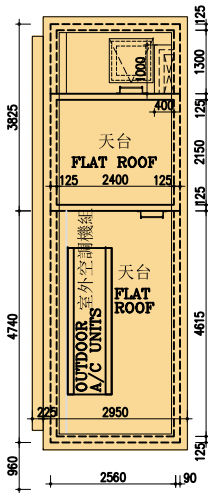
頂層天台 TOP ROOF
