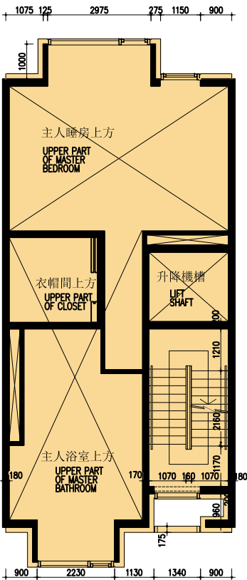
天台 ROOF AT LEV. +447.77
