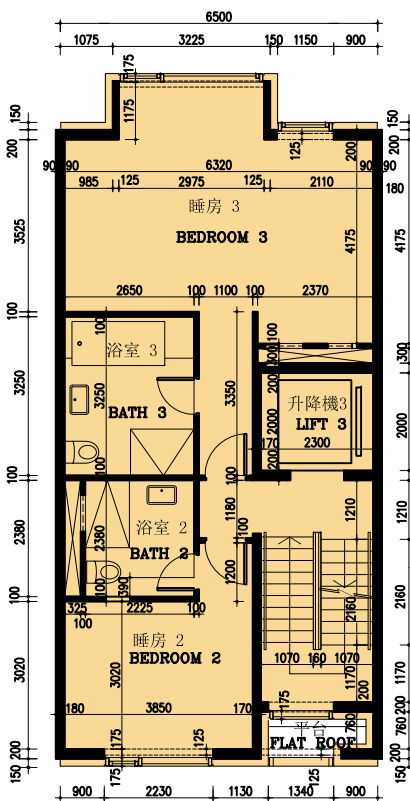
二樓 2ND FLOOR
