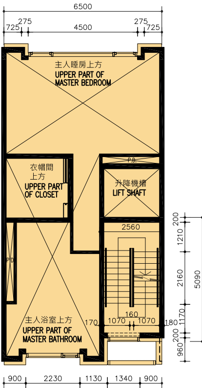
天台 ROOF AT LEVEL +447.77
