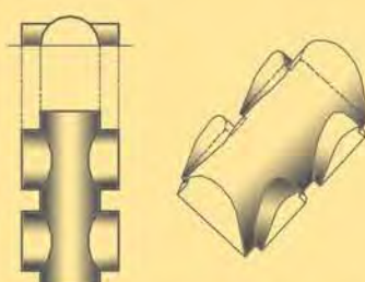
VOLTA A BOTTE CILINDRICA CON LUNETTE
