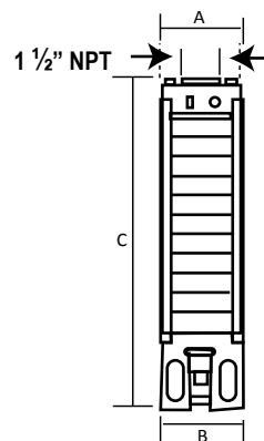
Acoplamiento NEMA 4"
