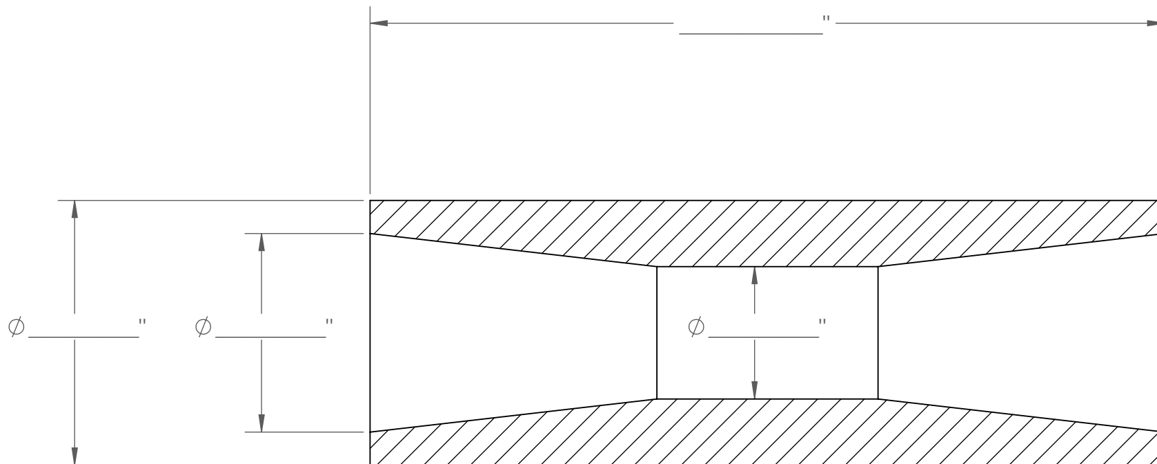
SECTION A-A SCALE 1 : 2
