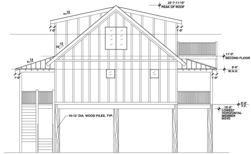
RIGHT ELEVATION
