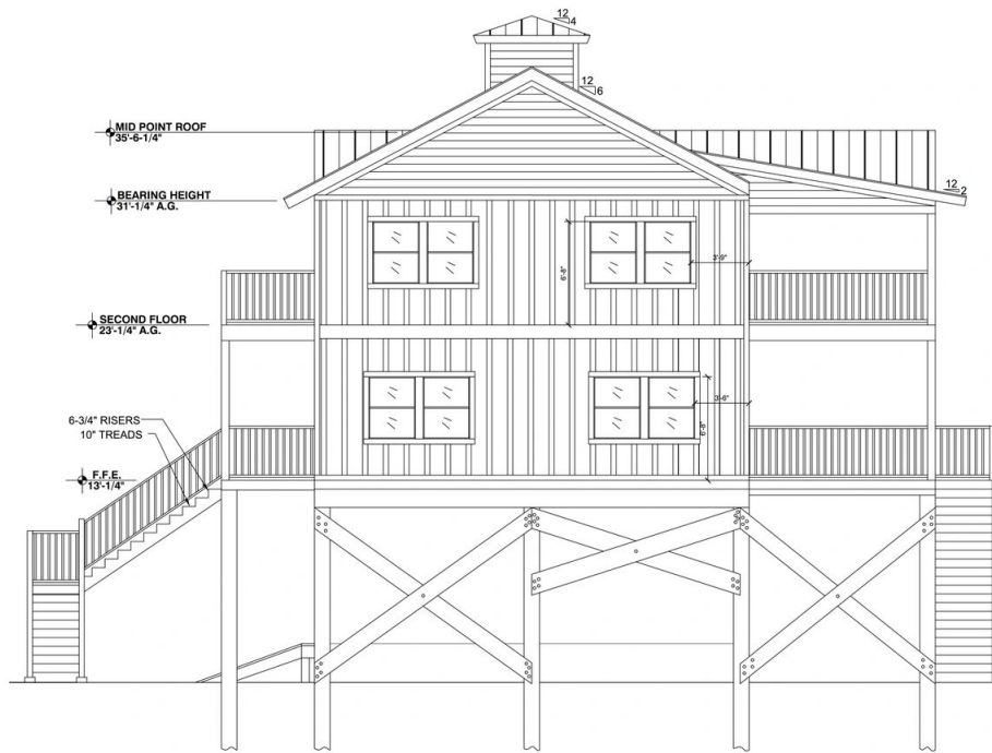
RIGHT ELEVATION
