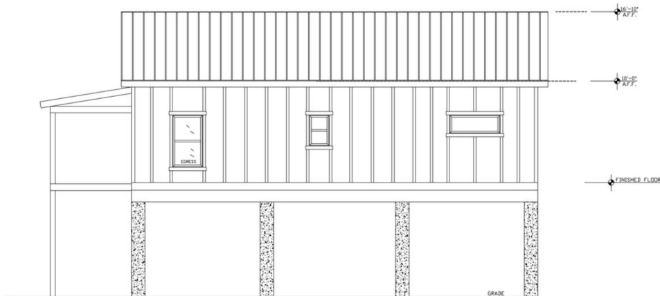
RIGHT ELEVATION
