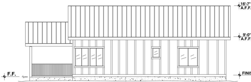
RIGHT ELEVATION
