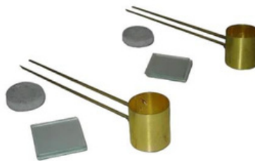
Le Chatelier Mould FI-305
