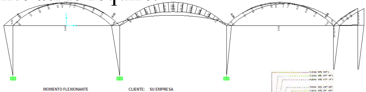
MOMENTO FLEXIONANTE
