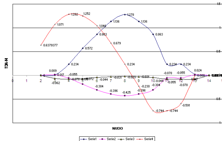
MOMENTO FLEXIONANTE
