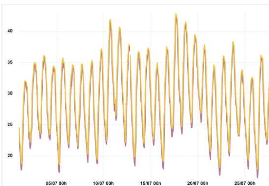
Gráfica de evolución de temperaturas (media, máxima y mínima) en julio de 2023.
