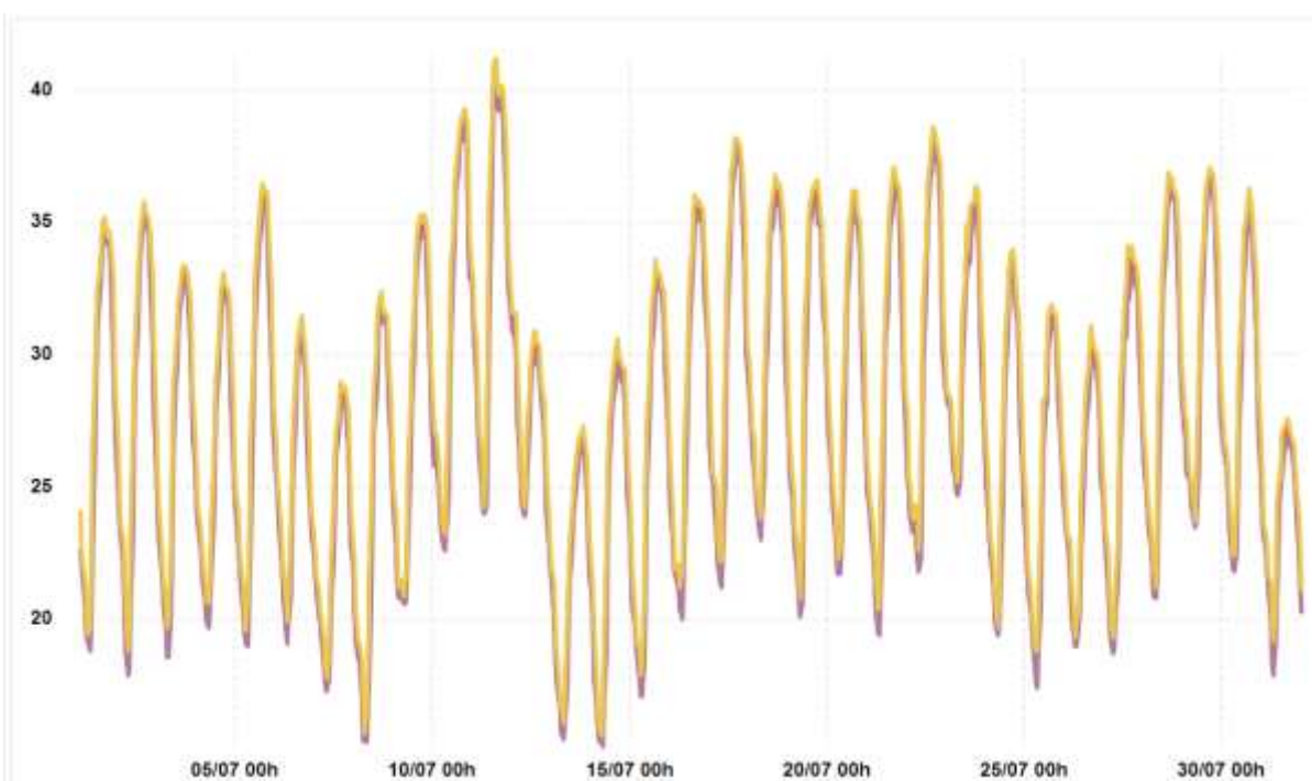
Gráfica de evolución de temperaturas (media, máxima y mínima) en julio de 2021.
