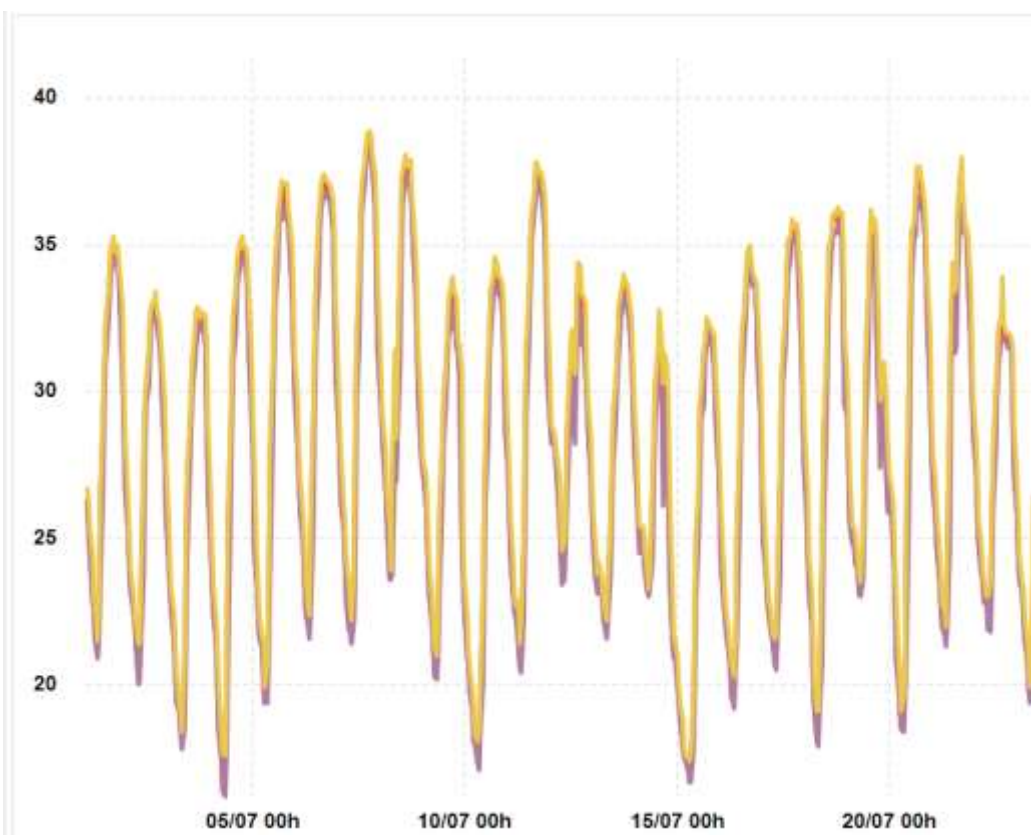
Gráfica de evolución de temperaturas (media, máxima y mínima) en julio de 2021.
