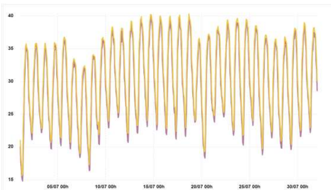
Gráfica de evolución de temperaturas (media, máxima y mínima) en julio de 2023.
