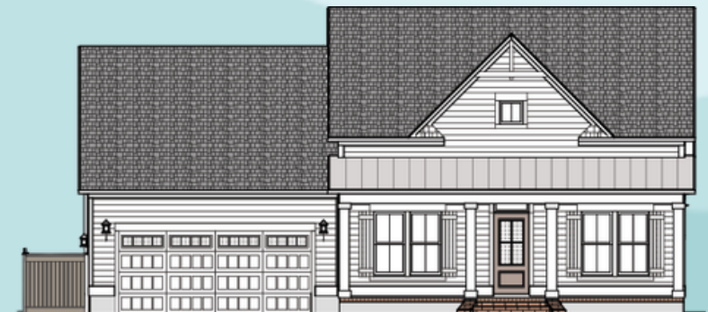
Elevation A
