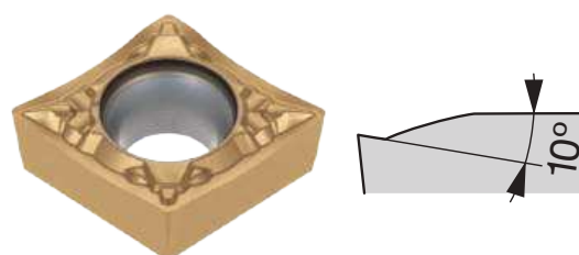
JS Chipbreaker
