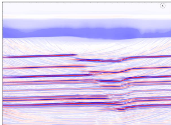
Perfil sísmico sintético de una modelo de fallas normales
