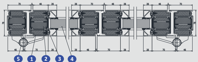
AS85 EI60 SISTEMA DE PUERTA DOBLE HOJA
