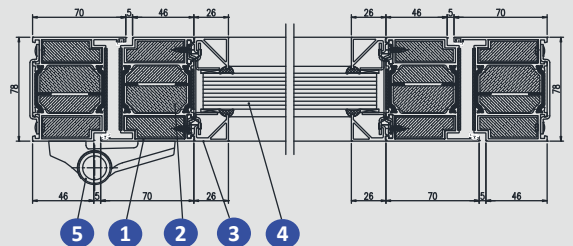
AS85 EI60 SISTEMA DE PUERTA DOBLE HOJA
