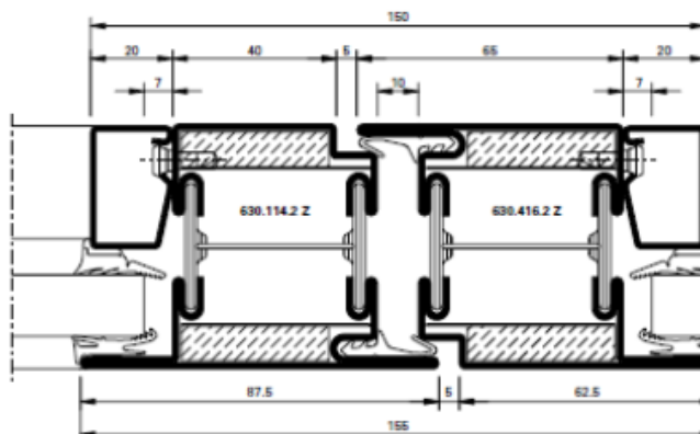
Detalle central de sección horizontal en puerta de 2 hojas Cotas en mm.
