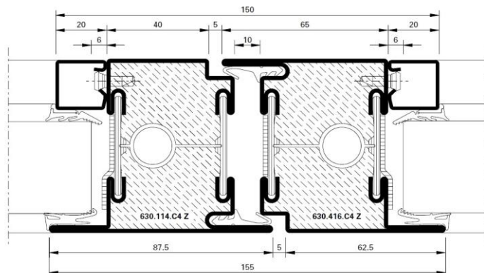
Detalle central de sección horizontal en puerta de 2 hojas Cotas en mm
