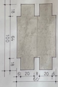
26 GLAVNI ZAMAJAC 1x3=3kom.
