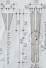
10) DEO KOTLJU DELA 2x3=6 kompleta
