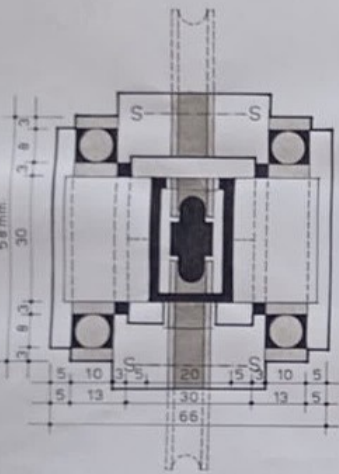
ČEONI PRESEK KLIZNO - ROTIRAJUĆE OSOVINE
