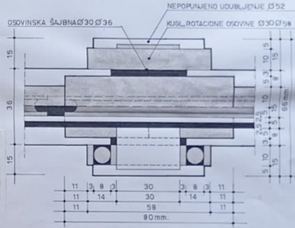
HORIZONTALNI IZGLED I PRESEK KLIZ. ROT. OSOVINE
