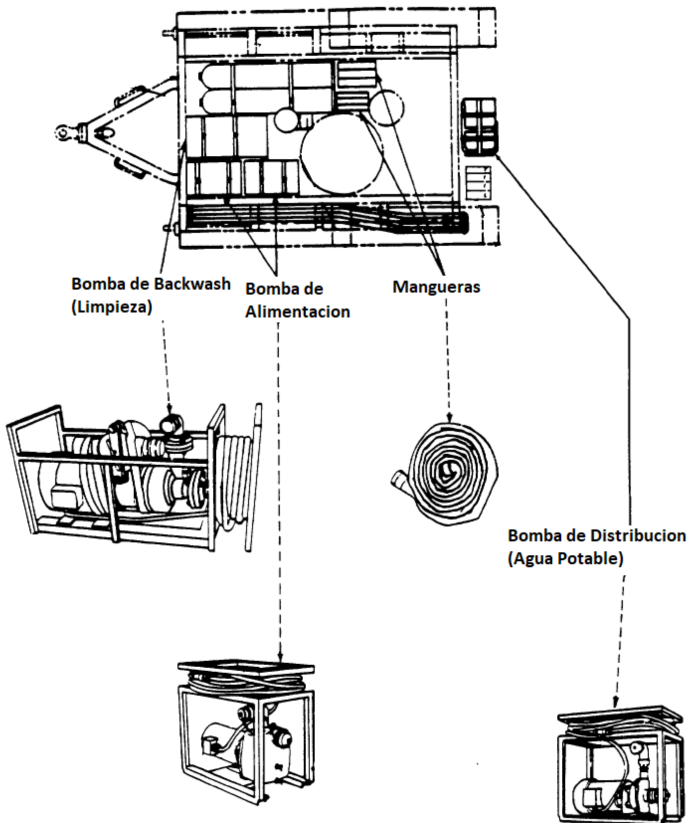
Figura 1. Componentes Planta Desaladora
