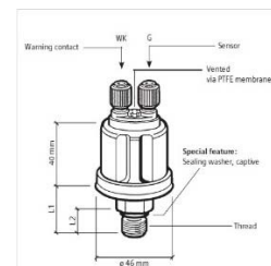
Sensor Switch de Presión 80PSI/5bar (E/RET) WC.25bar, M14X1.5
