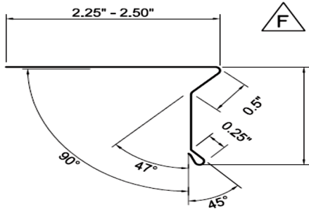
FT01 4.5" T-STYLE DRIP EDGE
