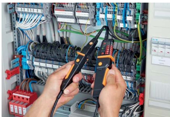
Medición de tensión en el armario de distribución.
