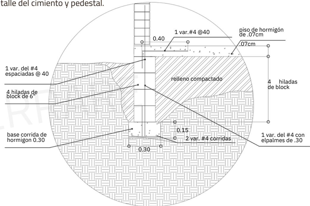
Detalle del cimiento y pedestal.
