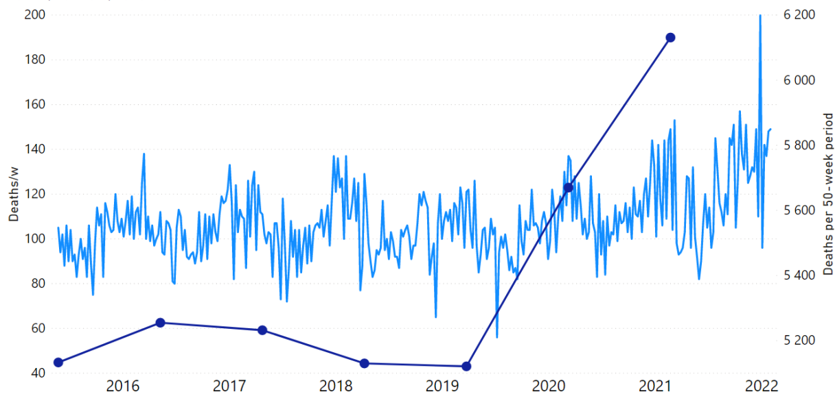
ACM/w, Vermont, 2015-2022
