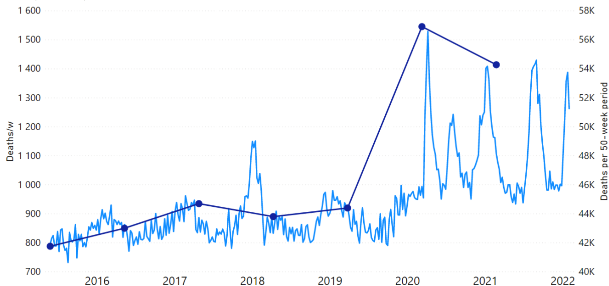
ACM/w, Louisiana, 2015-2022
