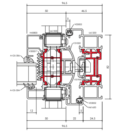
F82 LOCKING JAMB / C
