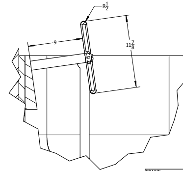
DETAIL B SCALE 0.20 : 1
