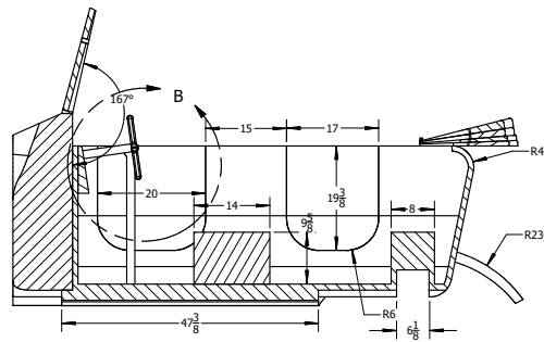
SECTION A-A SCALE 0.08 : 1
