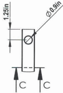
A DETAIL A N.T.S.
