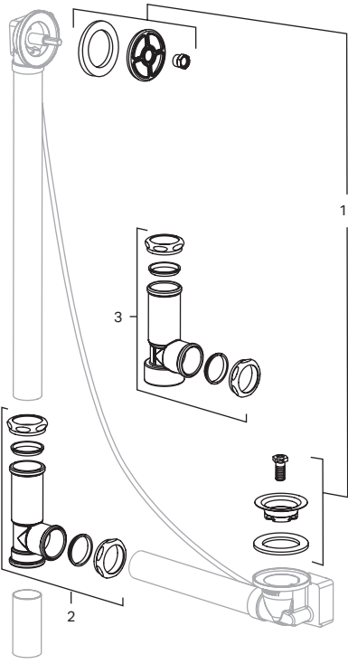
Tubular Brass
