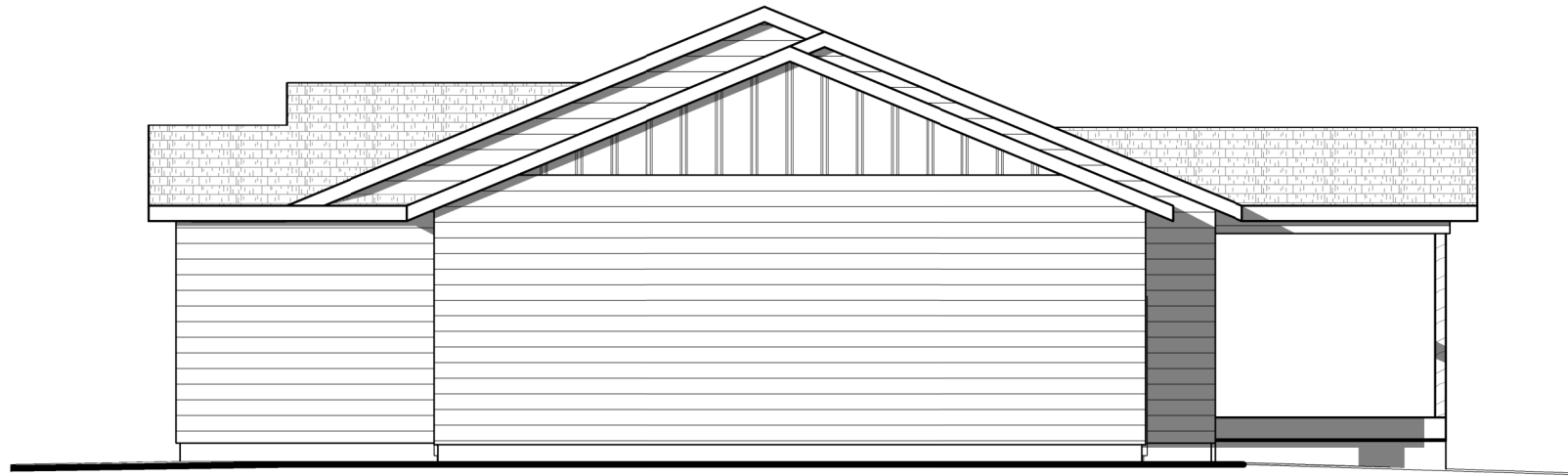
RIGHT ELEVATION
